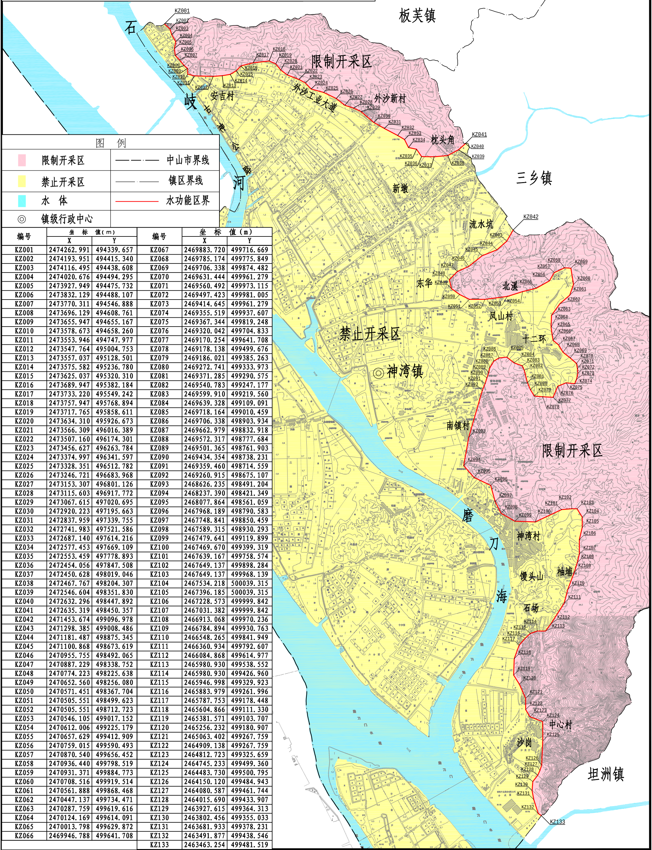
附图2-10 神湾镇浅层地下水功能区划
