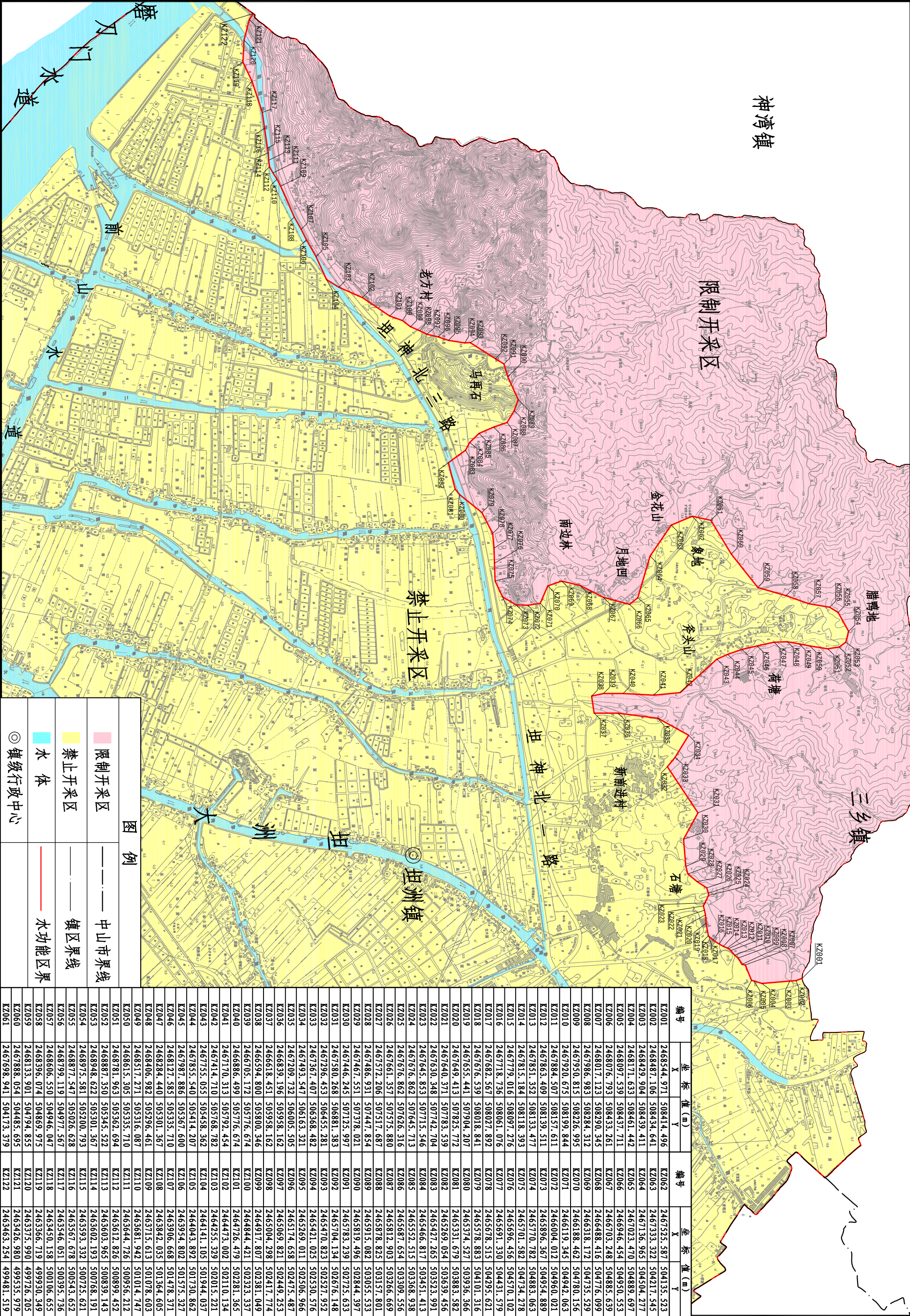
附图2-11 坦洲镇浅层地下水功能区划
