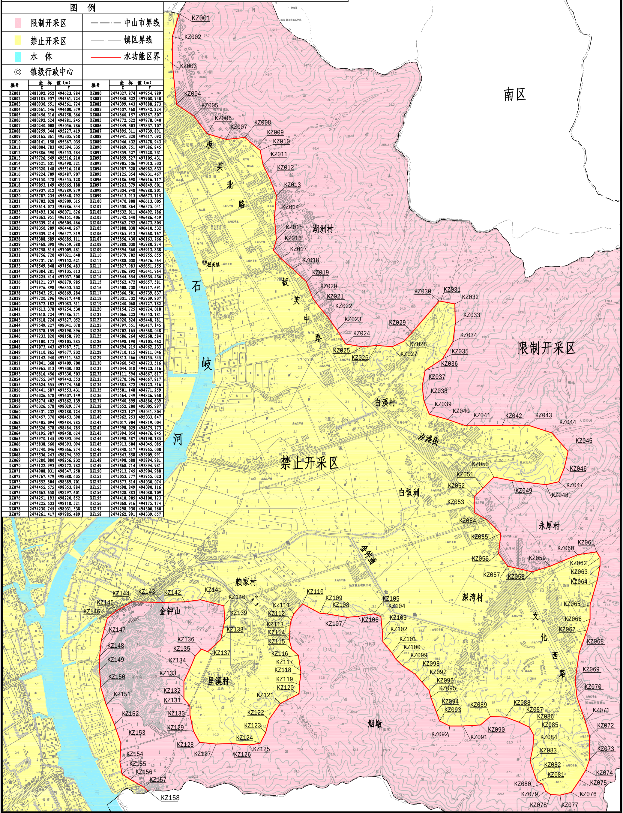
附图2-6 板芙镇浅层地下水功能区划
